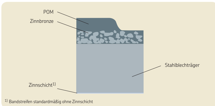
Querschnitt eines SKF POM Composite-Gleitlagers
