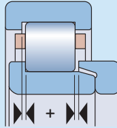
Axiale Lagerluft von Zylinderrollenlagern der Bauform NJ + HJ
