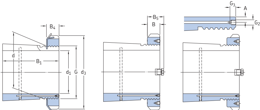
Ausführung OH .. H
