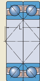
Lagerpaare in X-Anordnung
