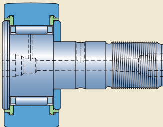
KR .. PPA, Größe ≥ 30
