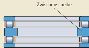
Lager mit Innenzentrierung
