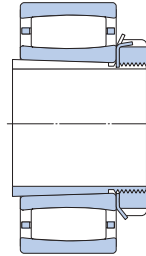
Lager auf Spannhülse der Standardausführung
