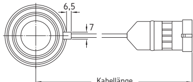
108A (mit Anschlussstecker AMP Superseal™)
