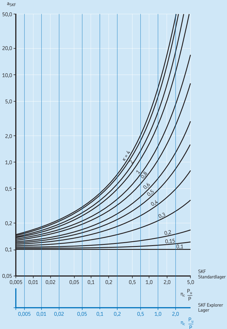
Lebensdauerbeiwert a_{SKF} für Axial-Rollenlager
