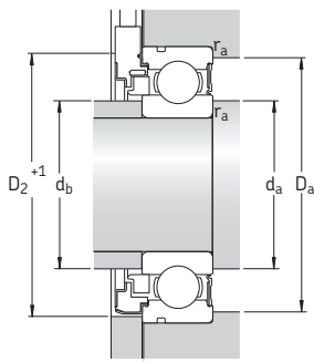
Bohrungsdurchmesser des Enddeckels \geq D_2 + 1 mm
