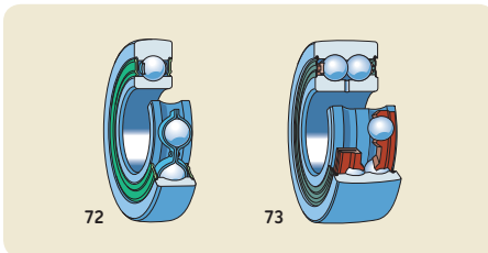
Laufrollen einreihig (72) zweiseihig (73)
