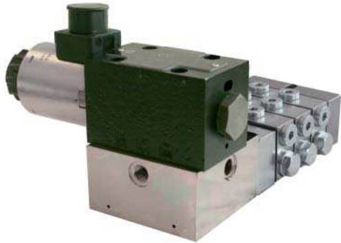
Mit 4/2-Wegemagnetventil
