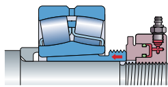
Matice HMV ..E našroubovaná na hřídeli při montáži stahovacího pouzdra
