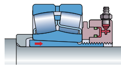
Matice HMV ..E při montáži ložiska na upínací pouzdro
