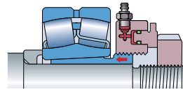
Matice HMV ..E a speciální zarážka při montáži stahovacího pouzdra
