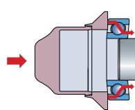
Montáž na hřídel s přesahem
