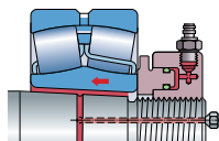
Matice HMV ..E při montáži ložiska na kuželovou úložnou plochu
