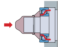
Montáž do tělesa s přesahem
